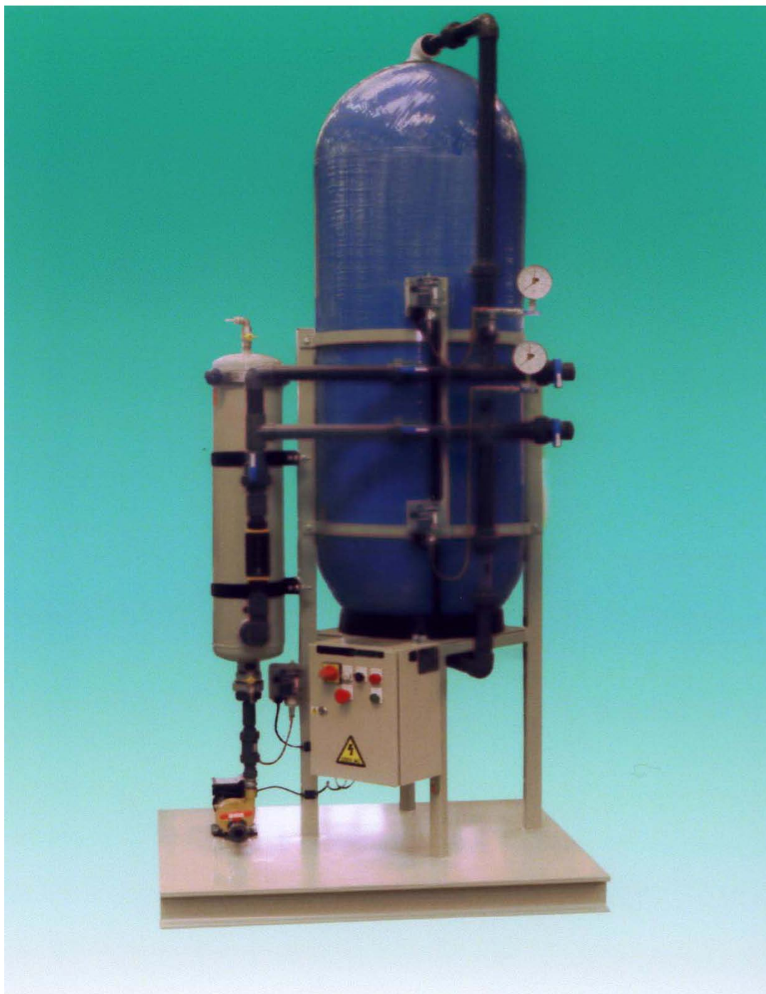
Węglowy zespół filtrujący S500C kompletny z filtrem koagulującym
